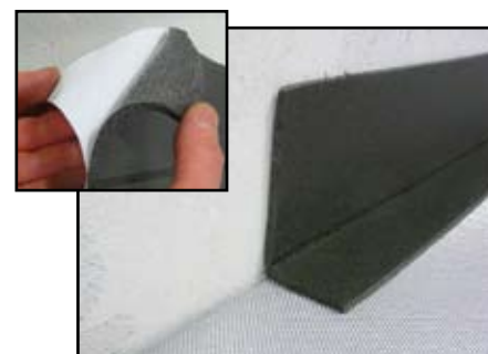
Verbinding tussen de muur en de insulit Bi+9 verwezenlijken met de zelfklevende Lfoam randstrook
